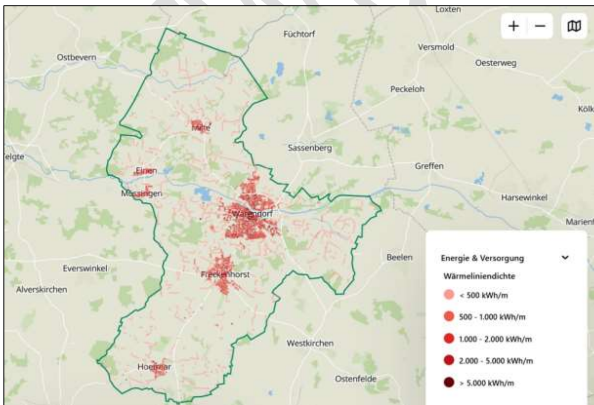
Abbildung 35: Straßenbezogene Wärmeliniedichte in Warendorf im Betrachtungsjahr 2022
