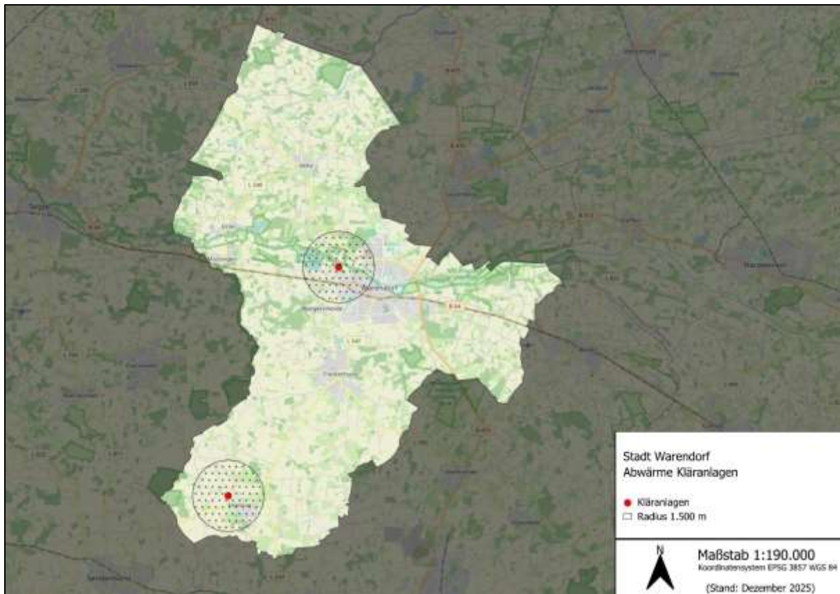
Abbildung 48: Kartografische Verortung der Kläranlage mit Abwärmepotenzial und Ermittlung relevanter Wärmebedarfe (1,5 km Radius)
